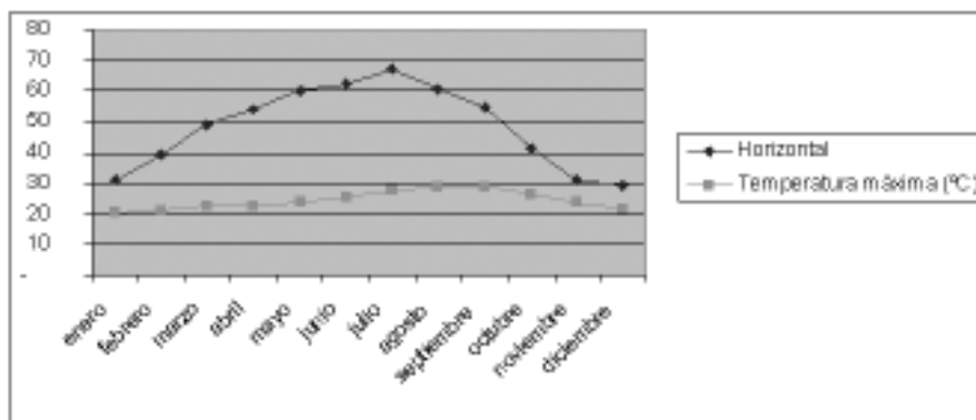
Figura 12. Evolución paralela de temperaturas máximas y radiación solar sobre cubiertas. Temperatura en ^{\circ}\text{C} y radiación sobre la superficie horizontal en 10^2 \text{ kWh/m}^2
