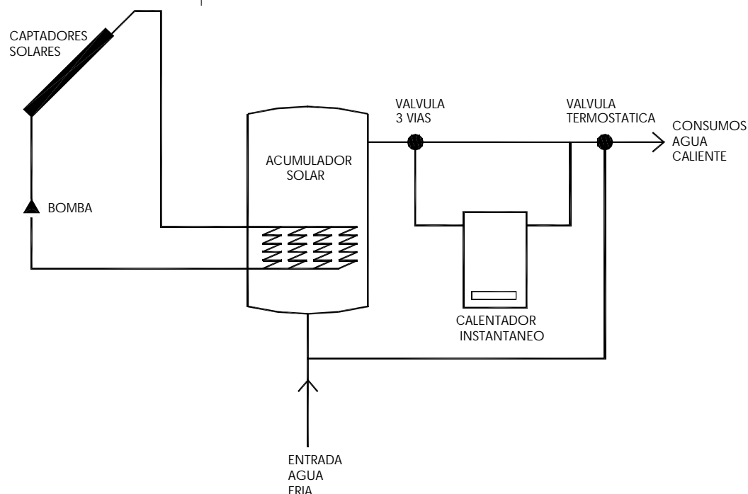
Figura 21. Esquema de equipo solar para agua caliente integrado con un calentador de gas auxiliar
