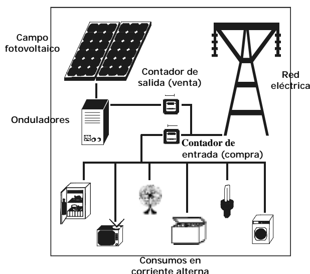
Figura 24. Esquema de instalación fotovoltaica conectada a la red eléctrica
