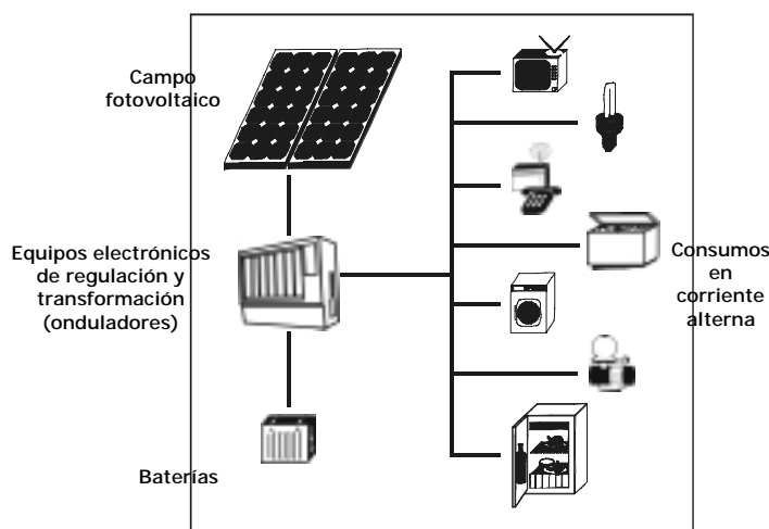
Figura 23. Esquema de instalación fotovoltaica autónoma
