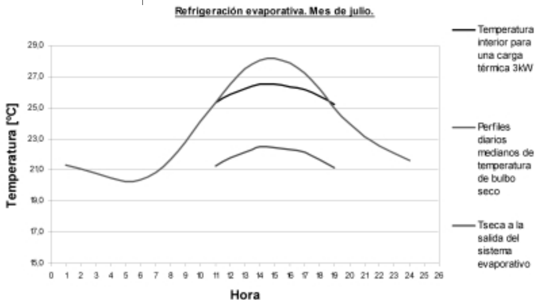
Figura 26. Evolución de temperatura interior utilizando un sistema evaporativo entre las 11 y las 20 h
