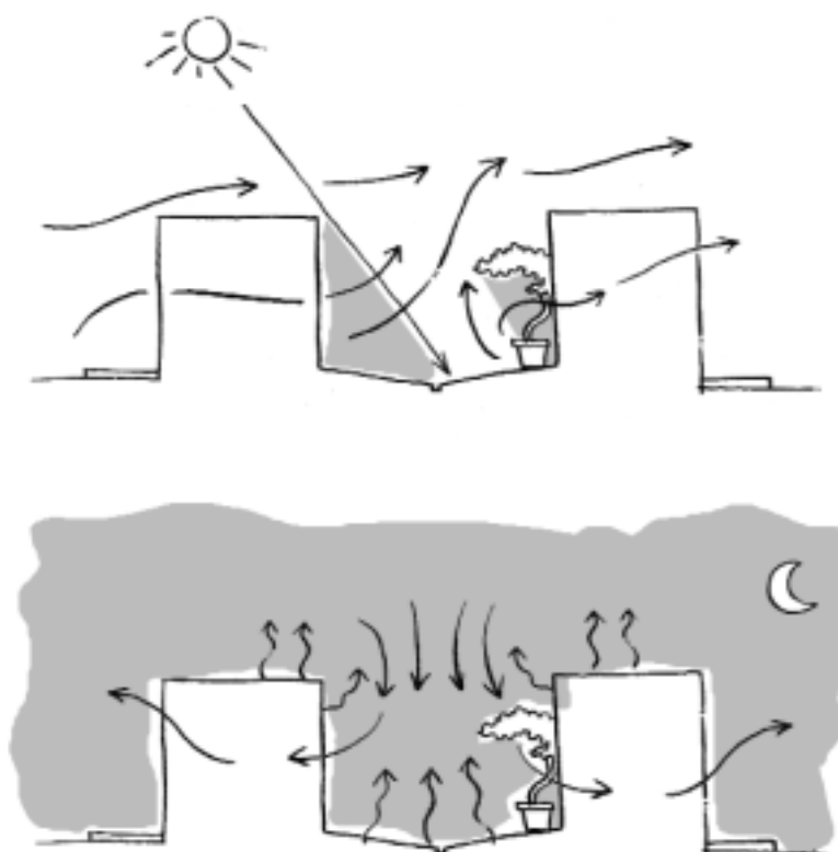
Figura 20: Comportamiento térmico de un patio interior de día y de noche
